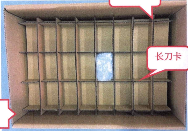
图二，每个气泡袋放 3 个 PA2633，1 格放 2 袋，共 6 个，每层 24 格放置 144 个，共 3 层，总计 432 个，同时在底层，顶层放 1 块隔板，中间 2 块，共 4 块。
